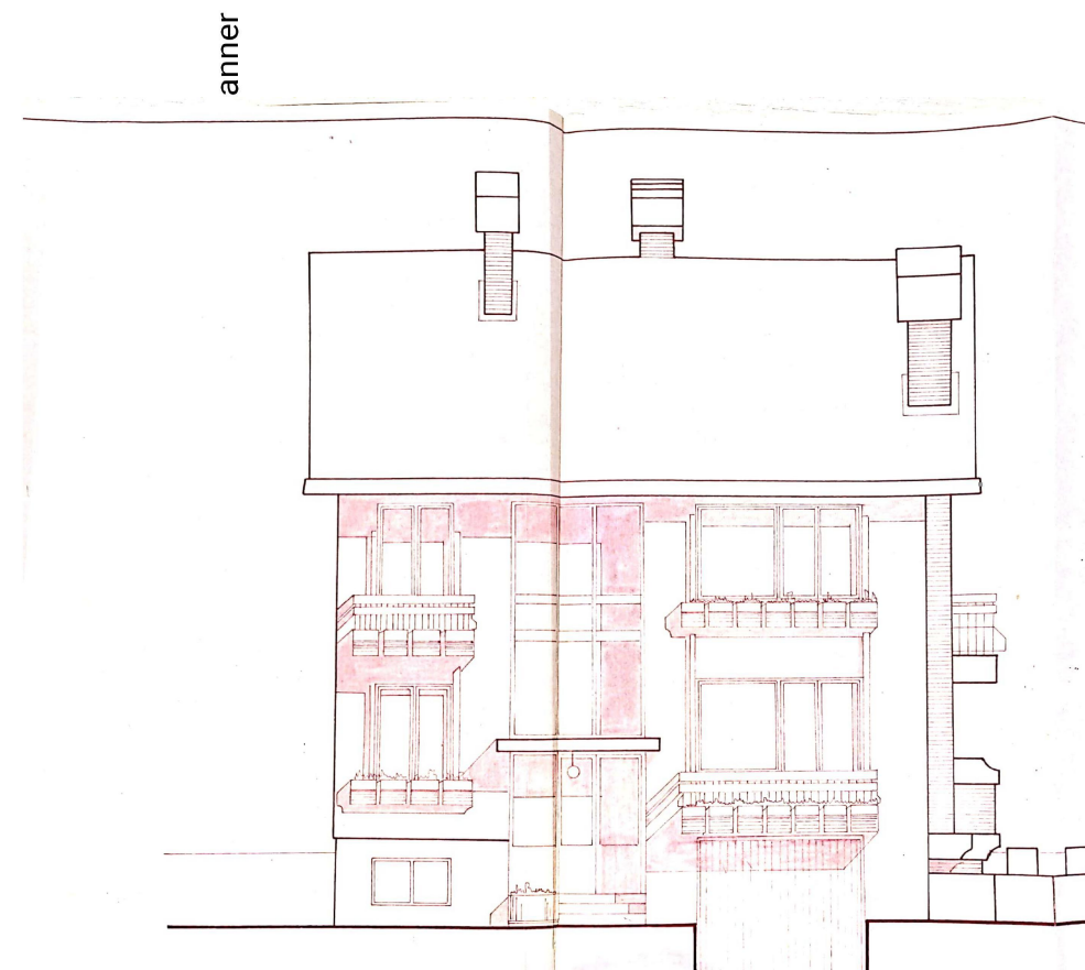
PREDNI IZGLED
