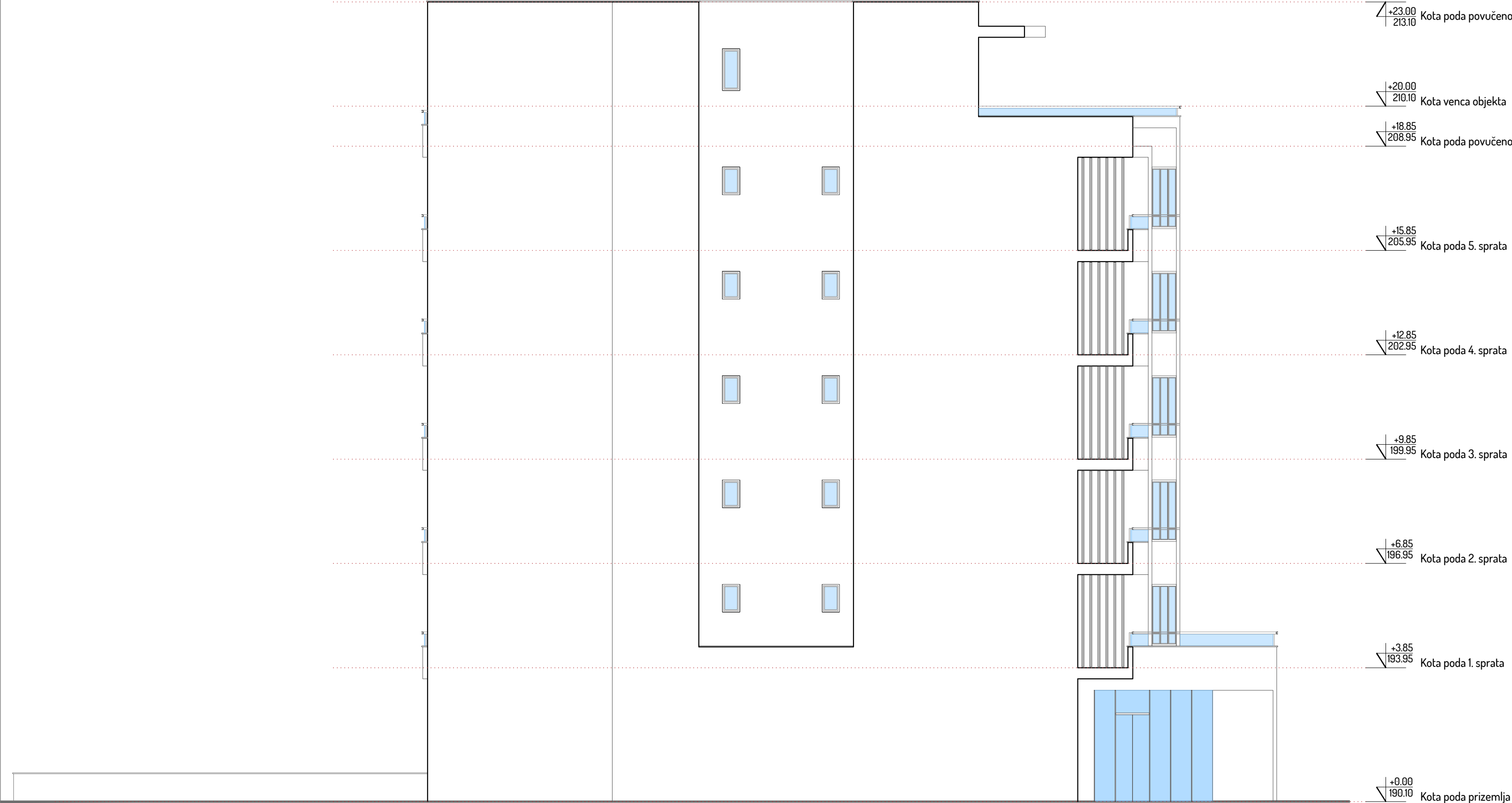
BOCNI IZGLED 2 R = 1:100
